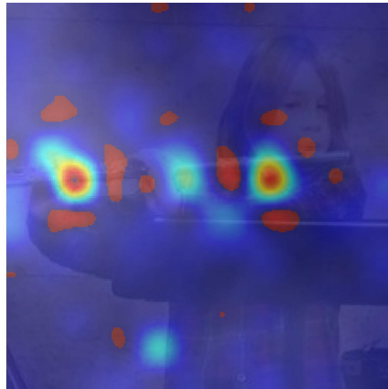
Ours(Fog)
